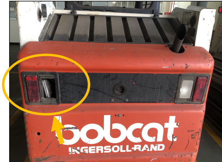
圖(三) 更換後尾燈總成
